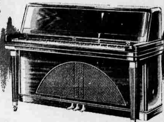
KNAPSODY MODEL
