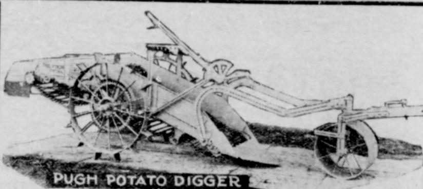
PUGH POTATO DIGGER
